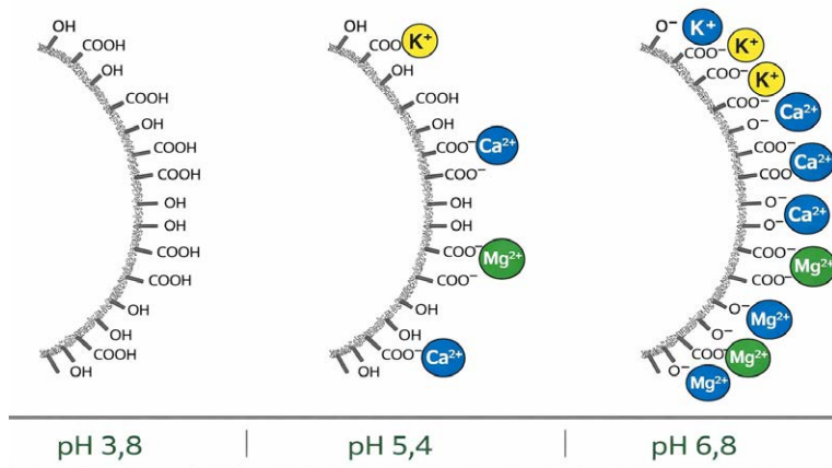
Rys.14. Wpływ pH na ładunek powierzchniowy koloidów próchnicznych.
