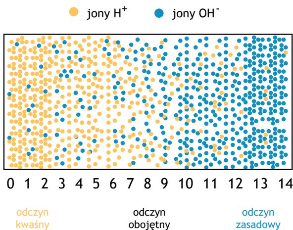
Rys. 1. Zasada funkcjonowania skali pH.
