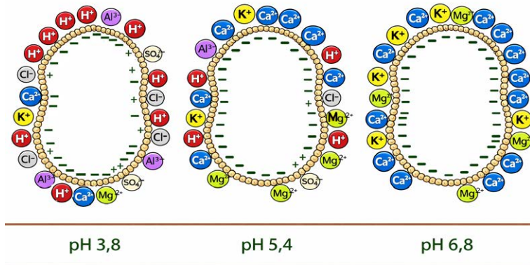
Rys.13. Wpływ pH na ładunek powierzchniowy niektórych koloidów mineralnych.
